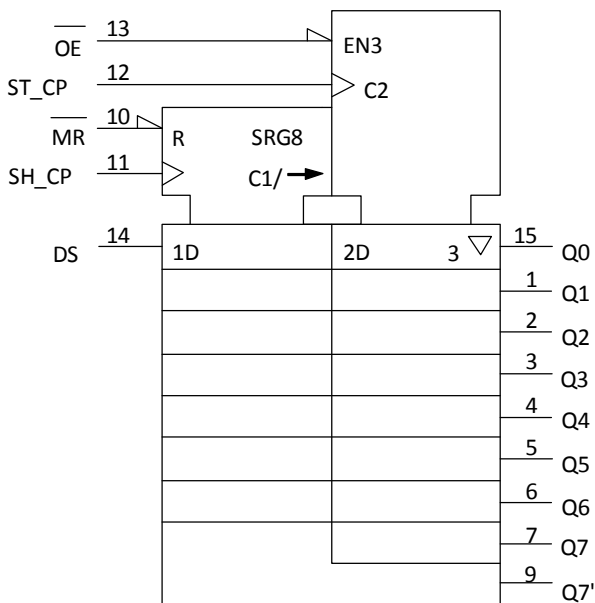
图 1 74HC595D功能图
