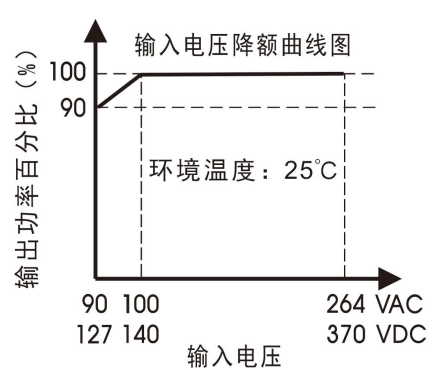
LOF350-20Bxx 输入电压降额
