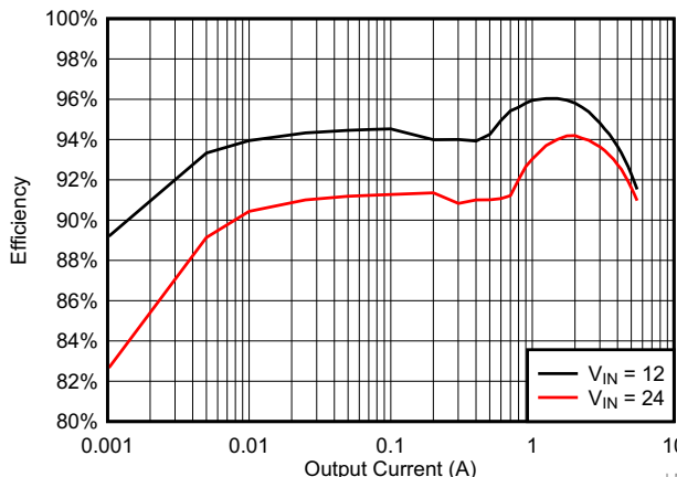
LMS3655-Q1 Efficiency: V_{OUT} = 5\text{ V}
