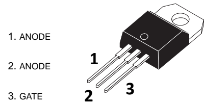
TO-220A (TO-220)
