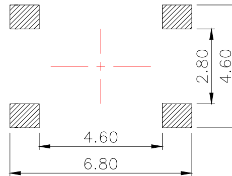
PCB.焊接图
