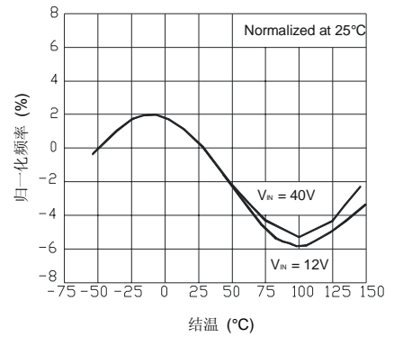
振荡器频率
