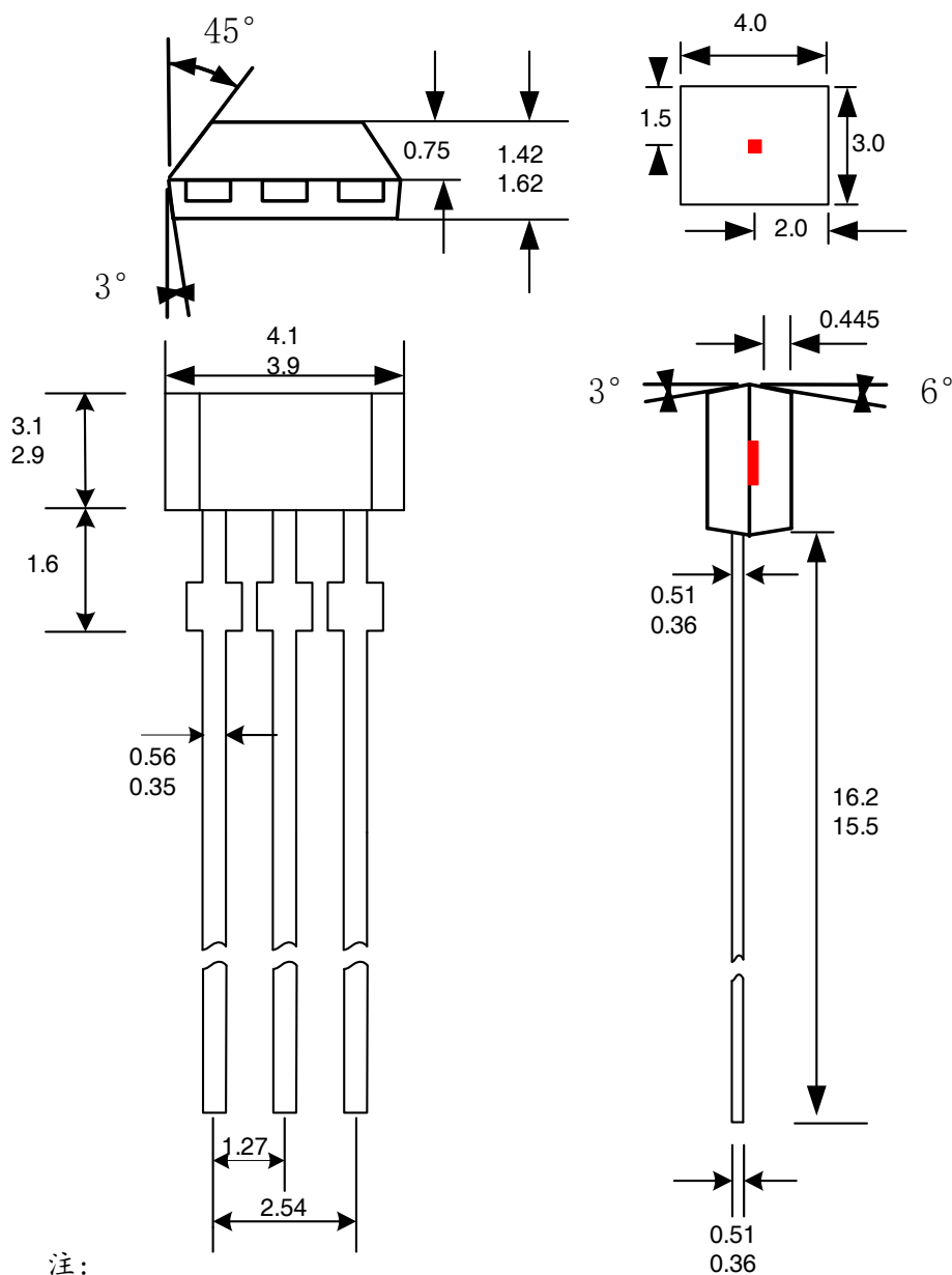
3-脚 UA 封装
