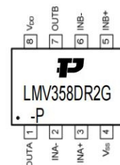
LMV358DR2G-P (SOP8)
