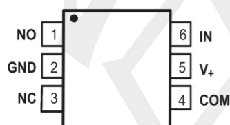
SOT363
