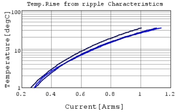
GJM1555C1H100JB01 Temp.rise 700MHz
