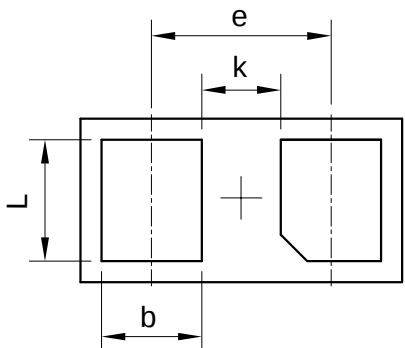
BOTTOM VVIEW
