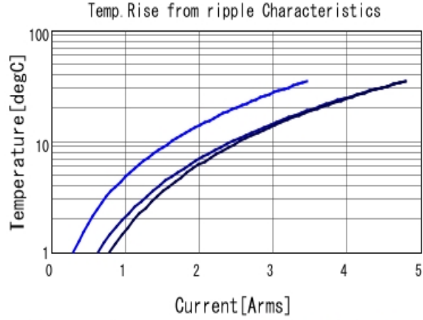
GRM188D70J106MA73 Temp. rise ■ 80kHz ■ 400kHz ■ 800kHz
