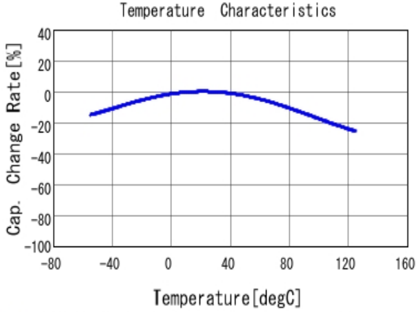
■ GRM188D70J106MA73 C-Temp. capchange, DCO. 0V, ACO. 2V rm
