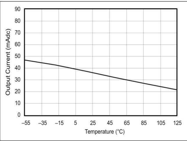
图2：温度 \propto 极限输出电流
