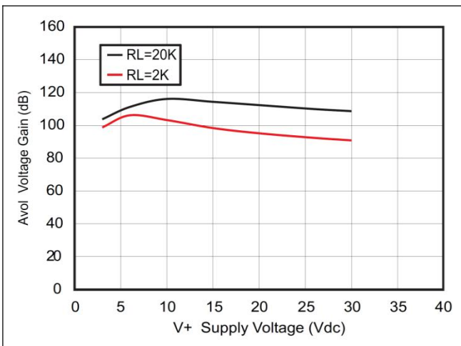
图5：电源电压 \propto 输出开环增益
