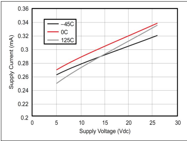
图1：电源电压 \propto 电源电流
