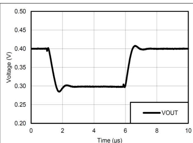
图8：电压跟随小信号响应（50pf）
