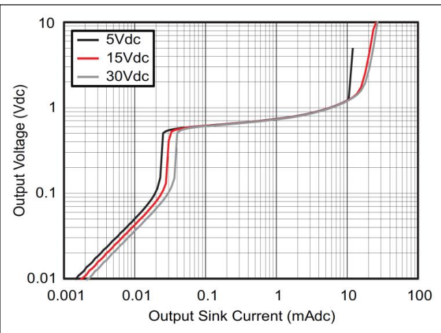
图4：极限灌电流 \propto 输出电压
