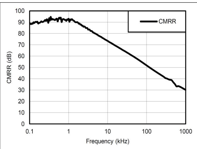
图6：频率 \propto 共模抑制比
