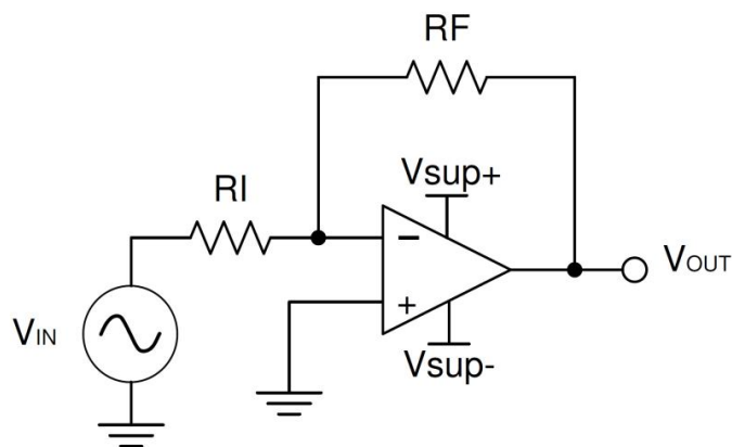
图1.应用原理图
