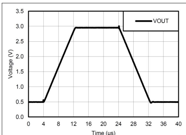
图7：电压跟随大信号响应（50pf）
