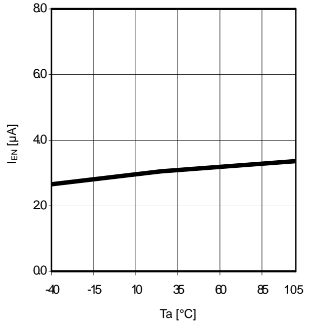
Figure 24. Ta-I EN
