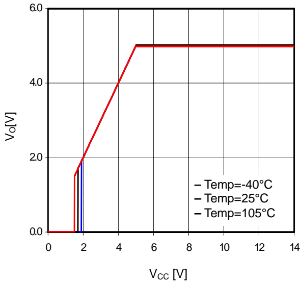
Figure 27. V_{CC}-V_o ( I_o=0 mA)
