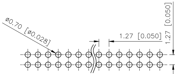
P.C.B Layout
