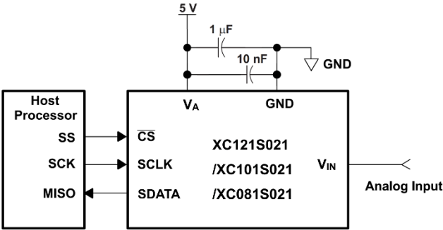
电路连接图
