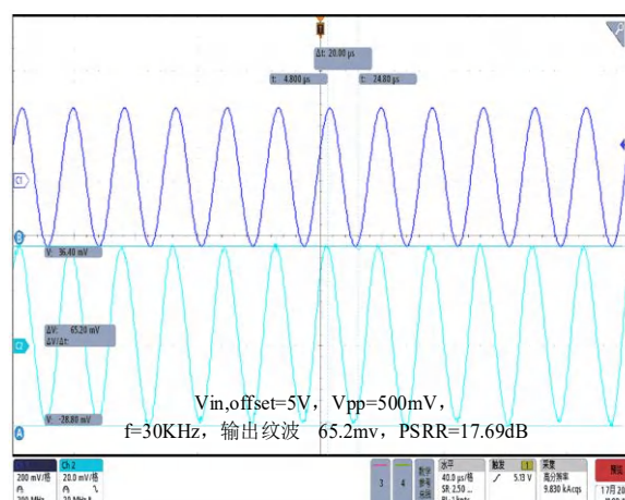
图6 纹波抑制比 ( f=30\text{KHz} )
