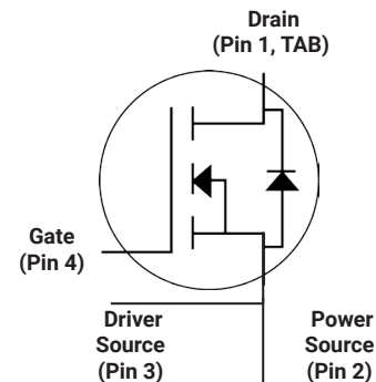
TO-247-4
