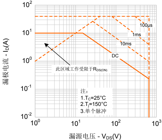
图9-4. 最大安全工作区域(SVF10N65S)
