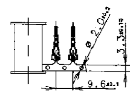
SEZ. C-C
