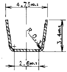
SEZ. C-C
