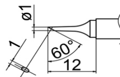
T12-C1 Shape-1C
