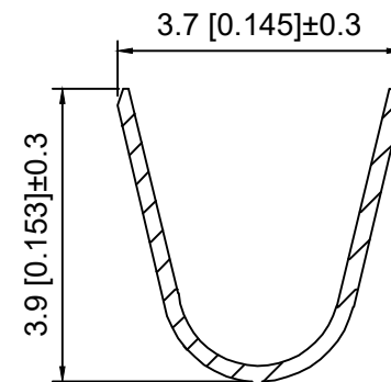
SEC:B-B
