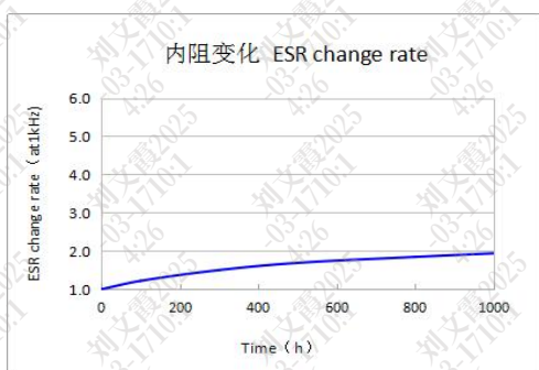
(3) 高温特性 High Temperature Life (at 5.5V, 65°C)
