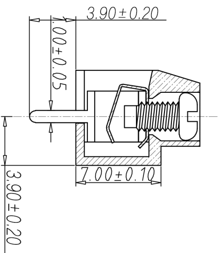
剖面图 A-A
