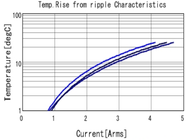
KCM55WR71J226MH01 Temp. rise ■ 50kHz ■ 100kHz ■ 300kHz
