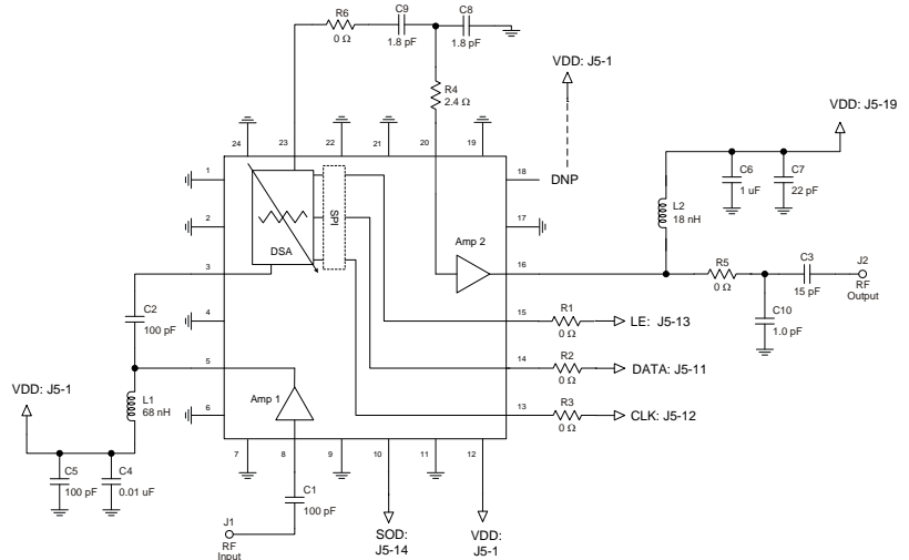
TQM879028 – 1805-1880 MHz
