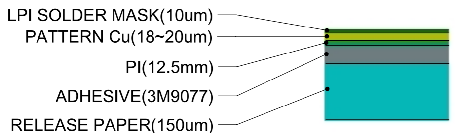
DETAIL A FLEX LAYER
