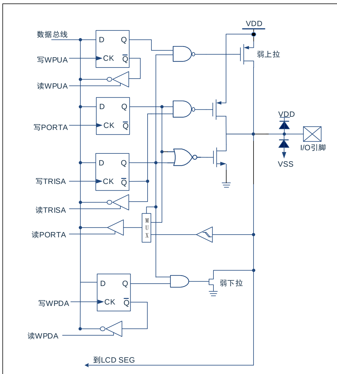
图 6-1: I/O 口结构图—PORTA
