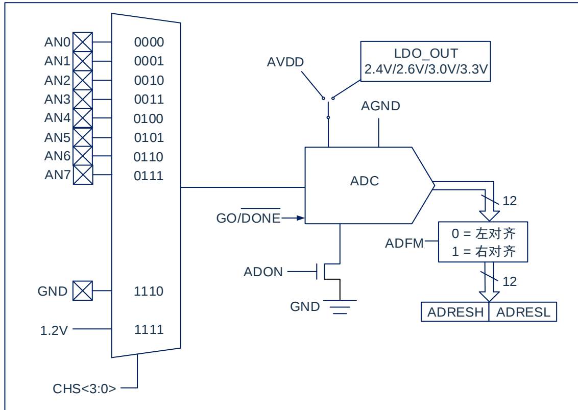
图 11-1：ADC 框图
