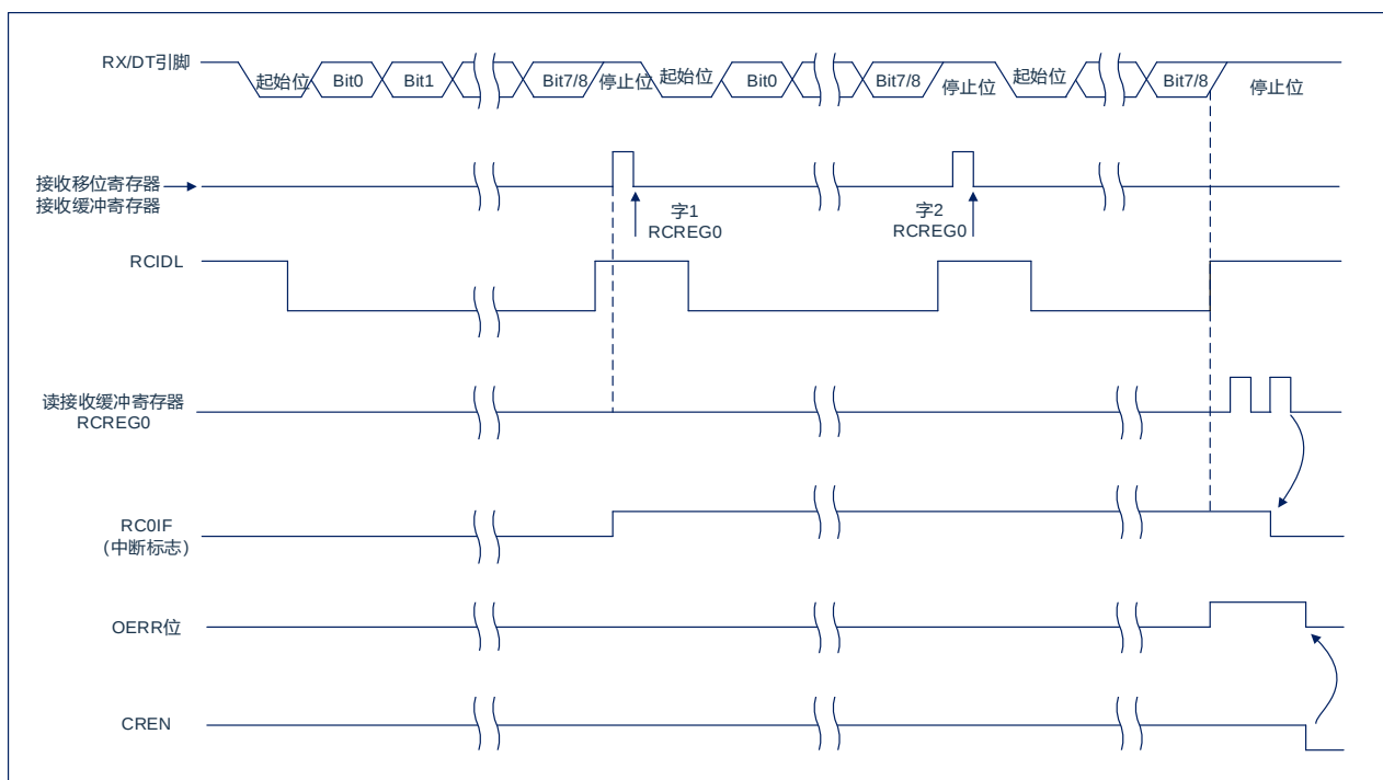
图 13-5: 异步接收
