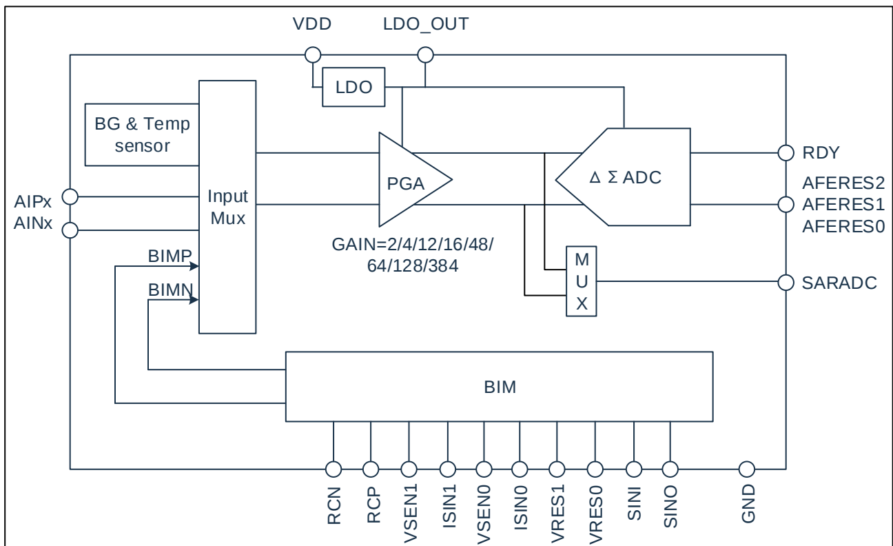
图 12-1: AFE 框图
