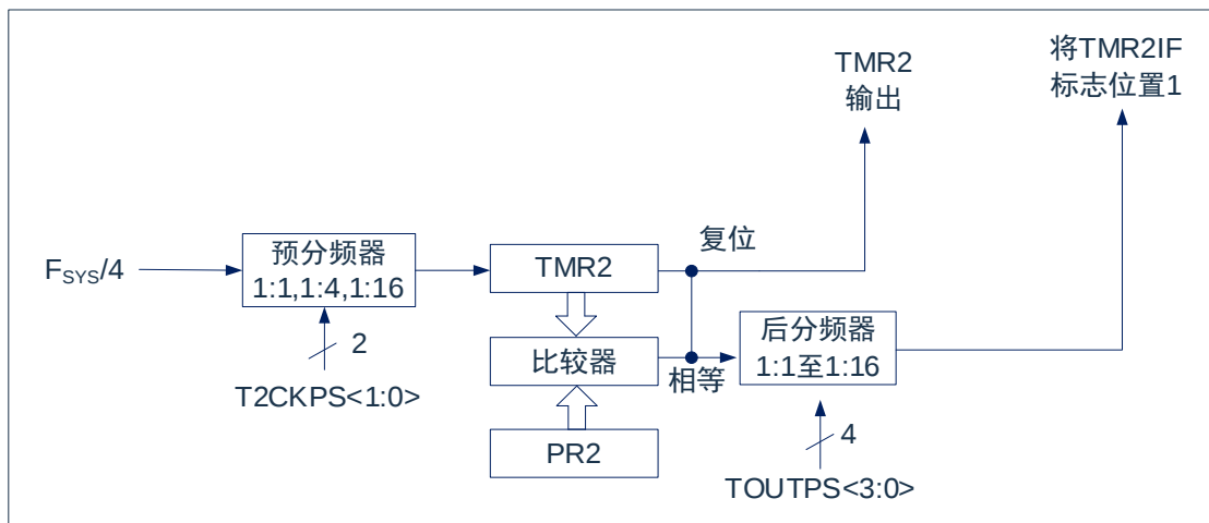
图 10-1: TIMER2 框图
