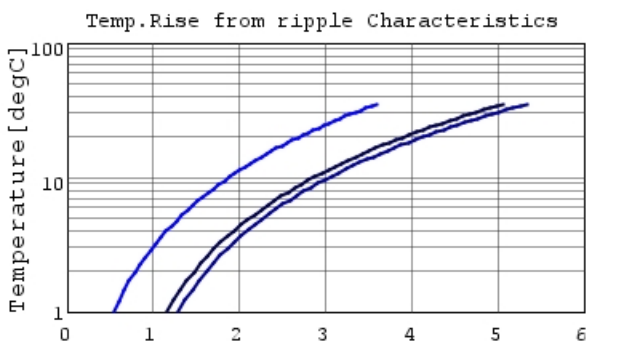
GRM31CB31E106KA75 Temp.rise — 80kHz
