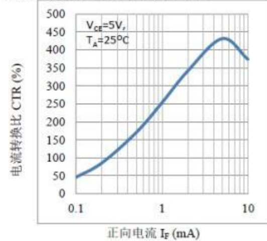
Fig.2 电流转换比 vs 正向电流曲线图
