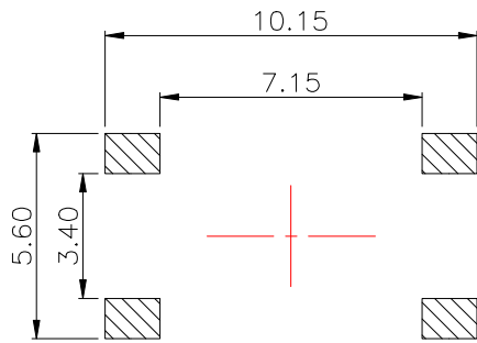
PCB.焊接图
