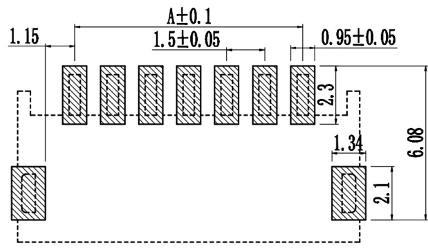
印制线路板
