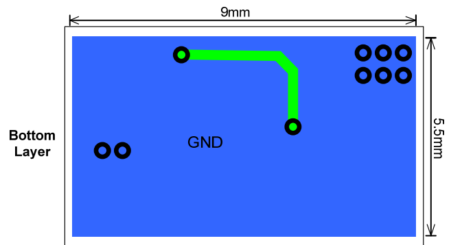
Figure 4— Bottom Layer
