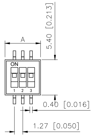
Dimensions (unit:mm)
