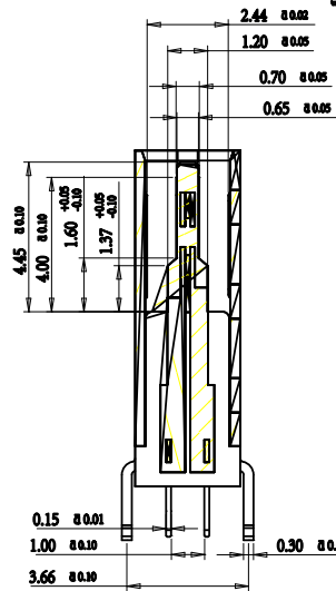
截面 1-1
