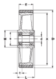
CUSCINETTO A RULLINI - ROLLER BEARING - ROLLENKORBLAGER - ROULEMENT À ROULEAUX - COJINETE A RODILLOS
