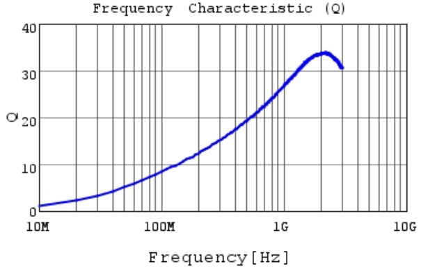
LQP03TN8N2H02 Q
