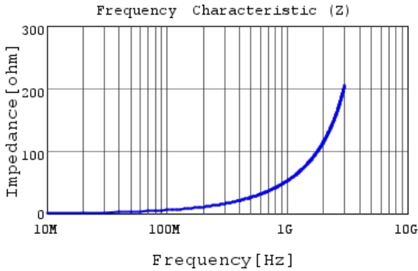
LQP03TN8N2H02 |Z|
