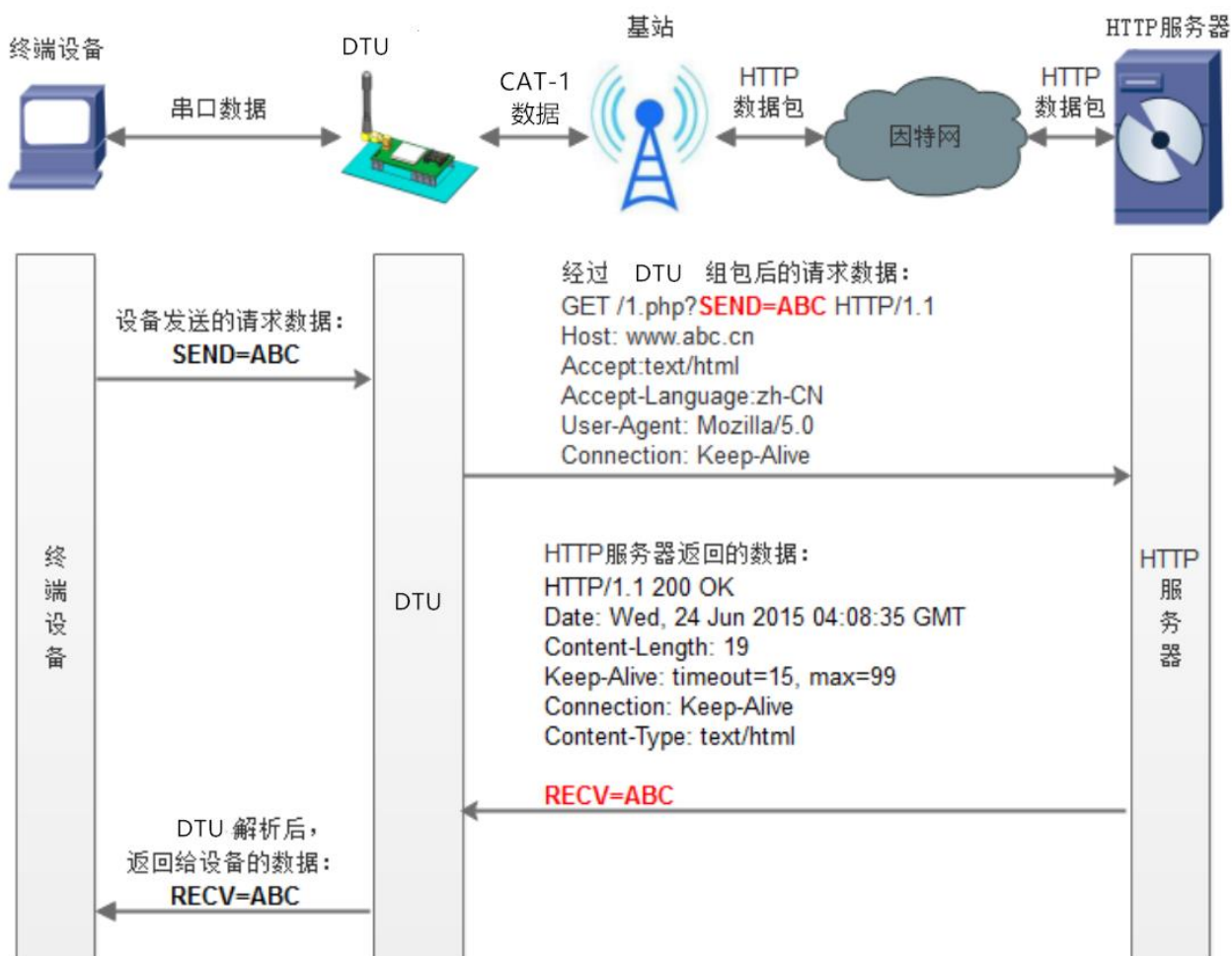
图7. HTTPD Client 模式
