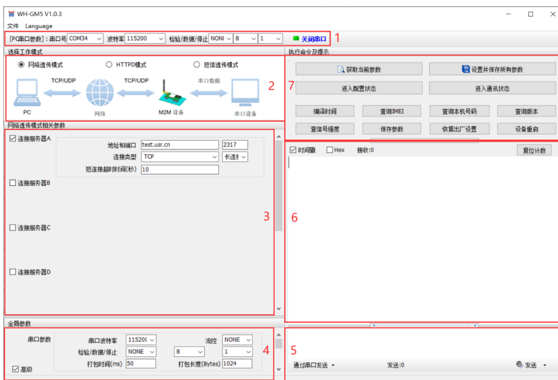
图23. 设置软件示意图
