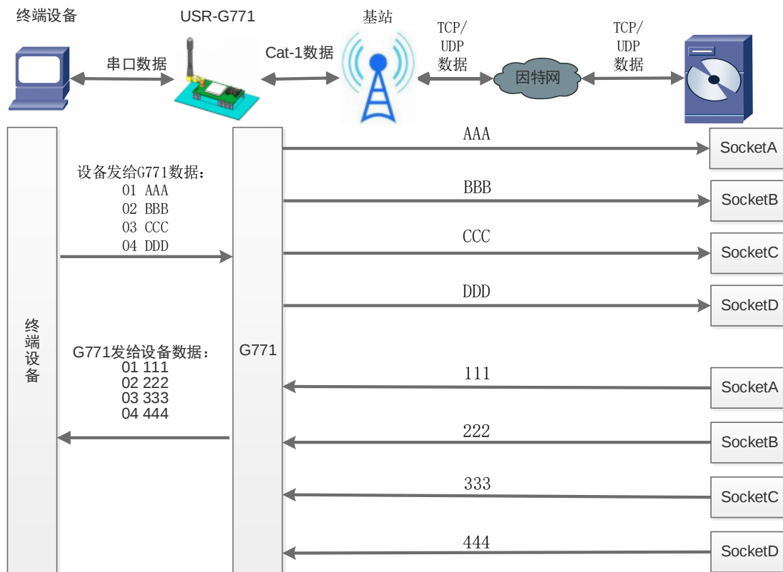
图13. 套接字分发协议示意图
