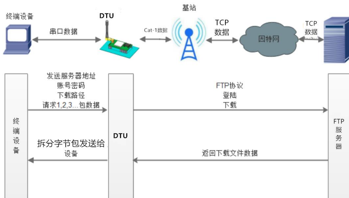
图18. FTP 他升级协议示意图
