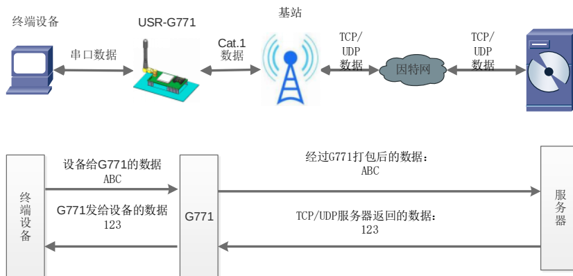
图5. 网络透传模式
