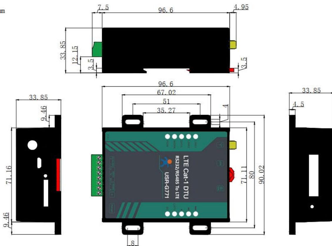
图2. USR-G771 尺寸图
