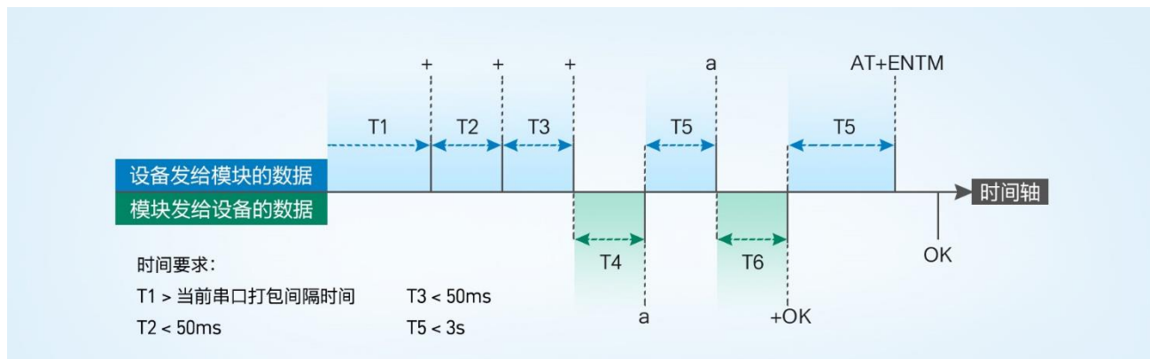
图26. 切换指令模式时序
