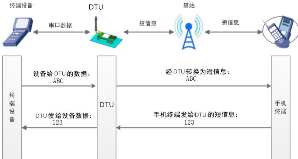
图9. 短信透传模式图
