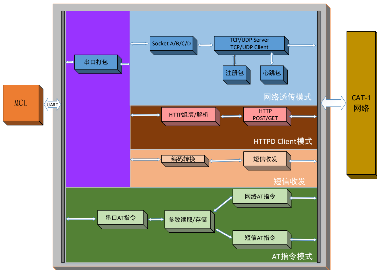
图4. 功能框图
