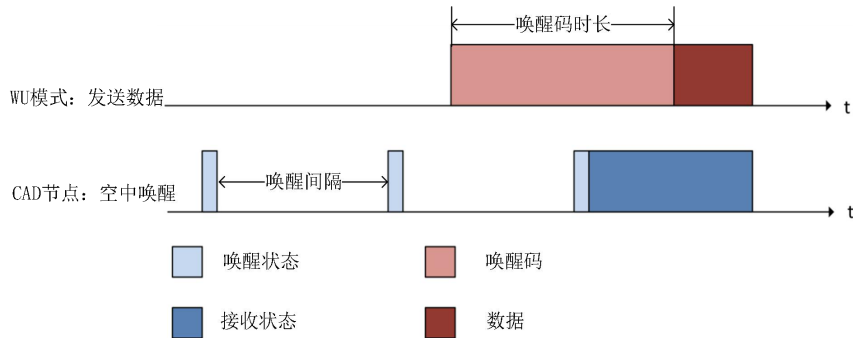
图 25 WU 模式唤醒 CAD 节点工作流程
