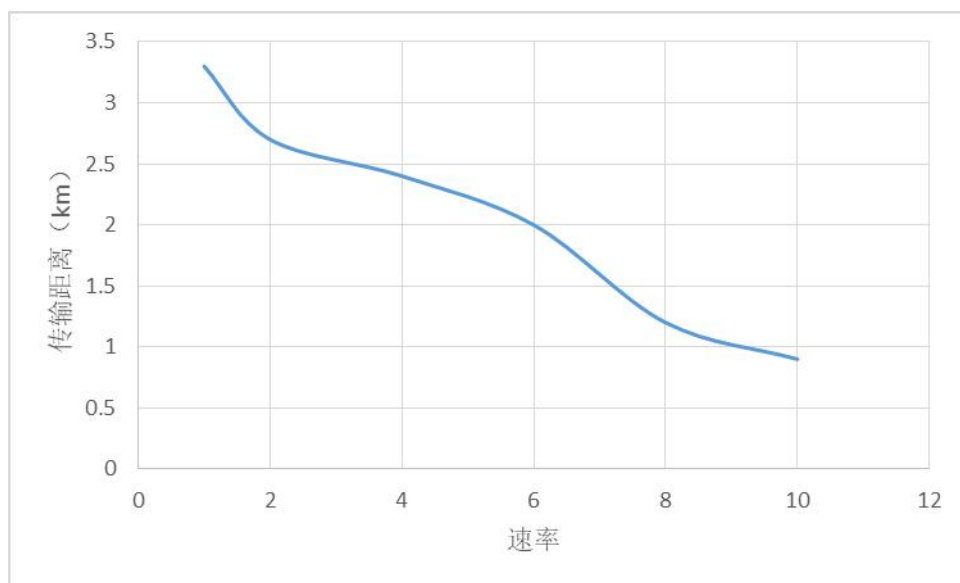
图 10 速率与传输距离曲线图
