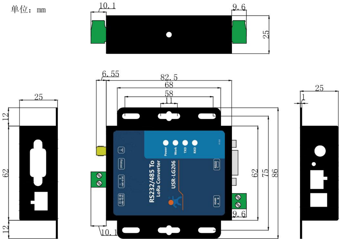
图 6 外观尺寸图
