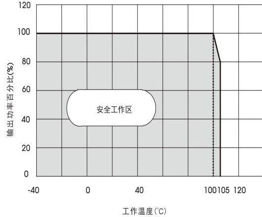
温度降额曲线
