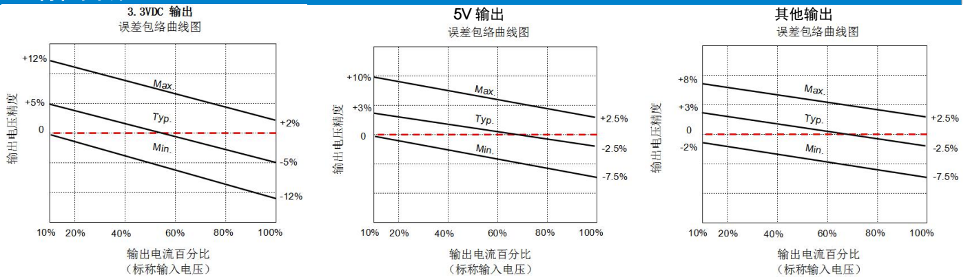
图 1 温度降额曲线
