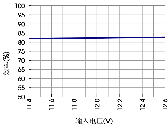
图 12 (输入电压与效率关系曲线)
