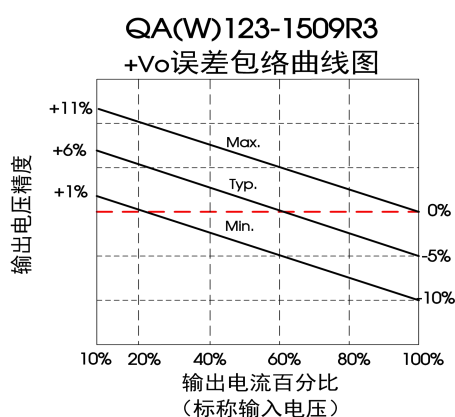
图 2 (主路误差包络曲线)
