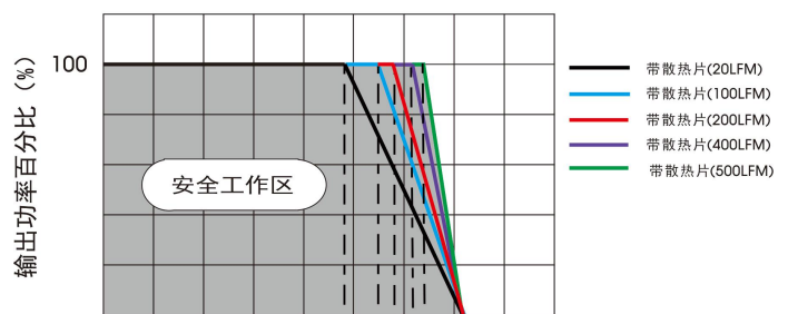
温度降额曲线图
