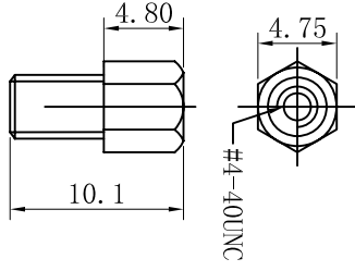
螺丝示意图
