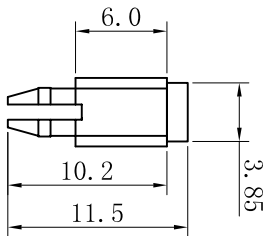
铆钉示意图
