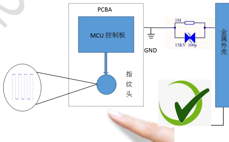
图（2） 接地问题正确示意图
