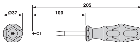
尺寸图
