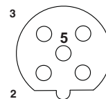
M12孔式连接器引脚分配，5芯，B编码，插座侧
