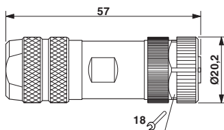
尺寸图
