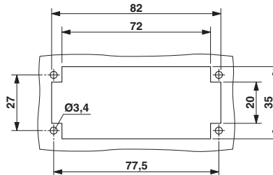
不使用外壳时的安装开口
