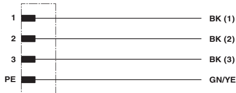
电路图
