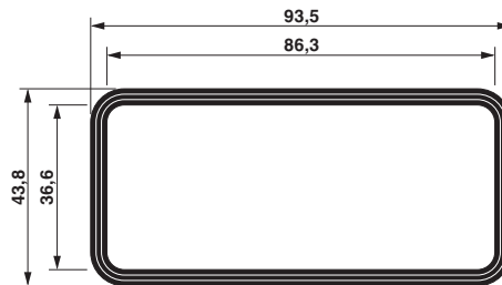
尺寸图
